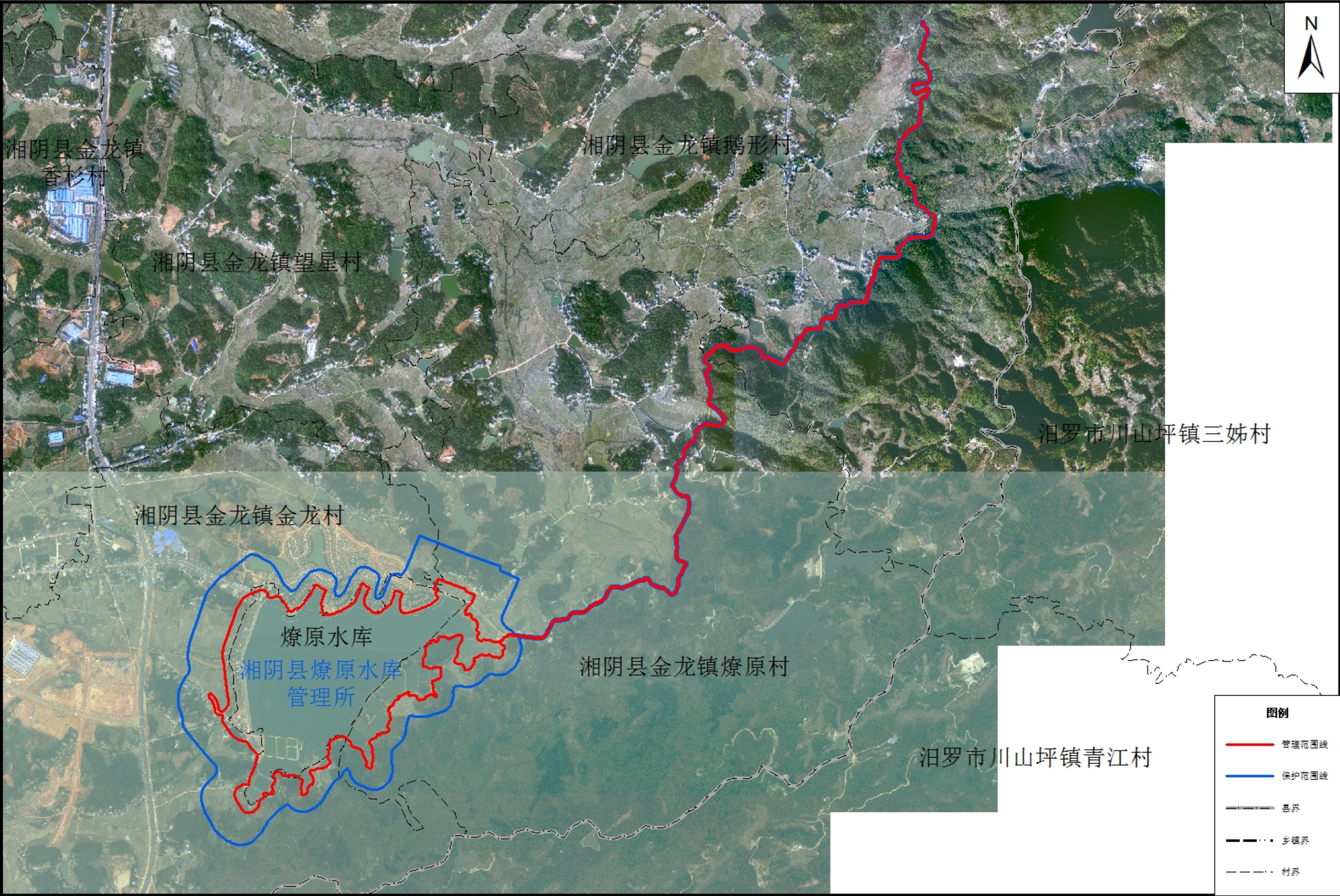
燎原水库管理与保护范围划界成果示意图
