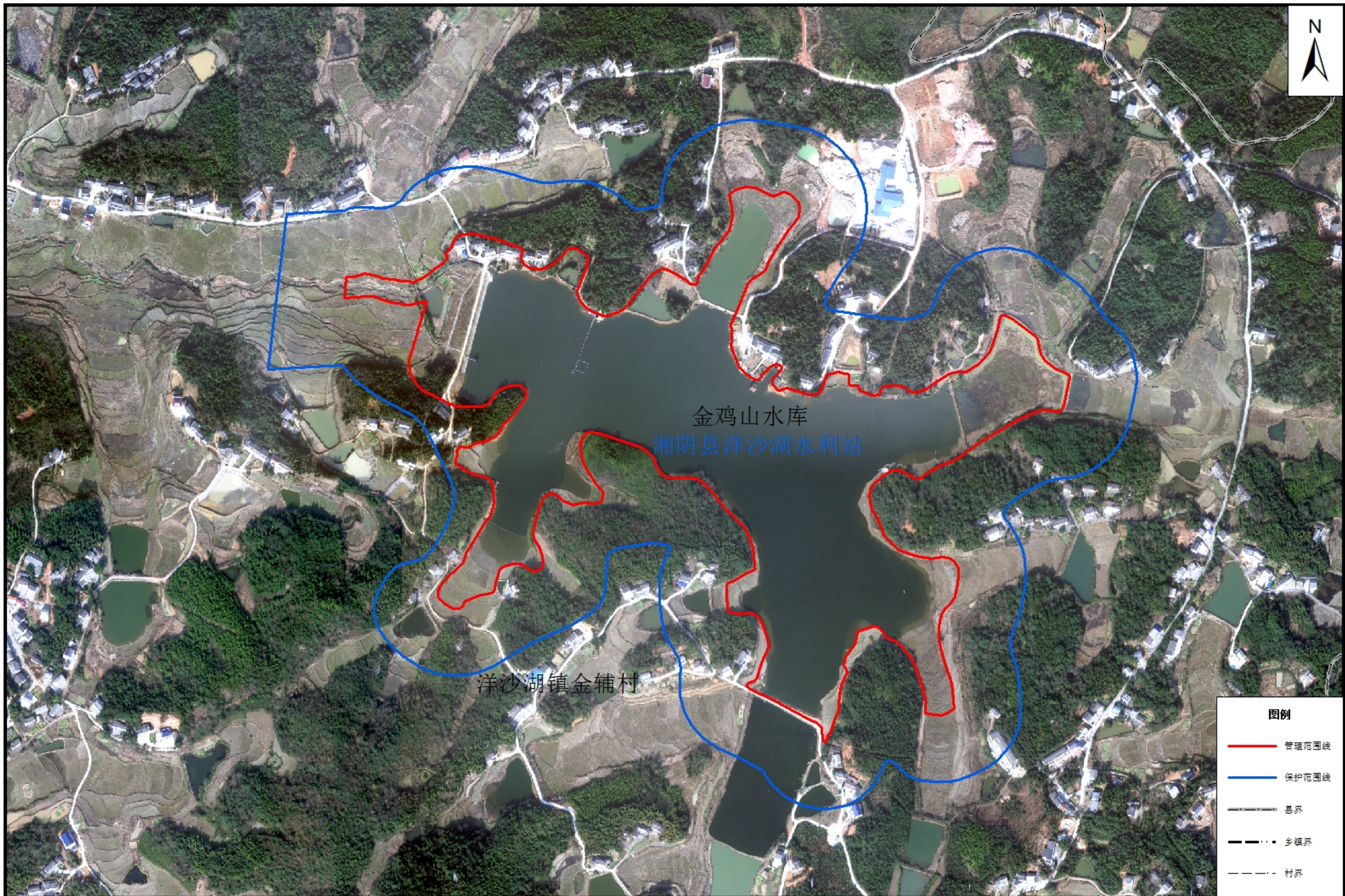
金鸡山水库管理与保护范围划界成果示意图
