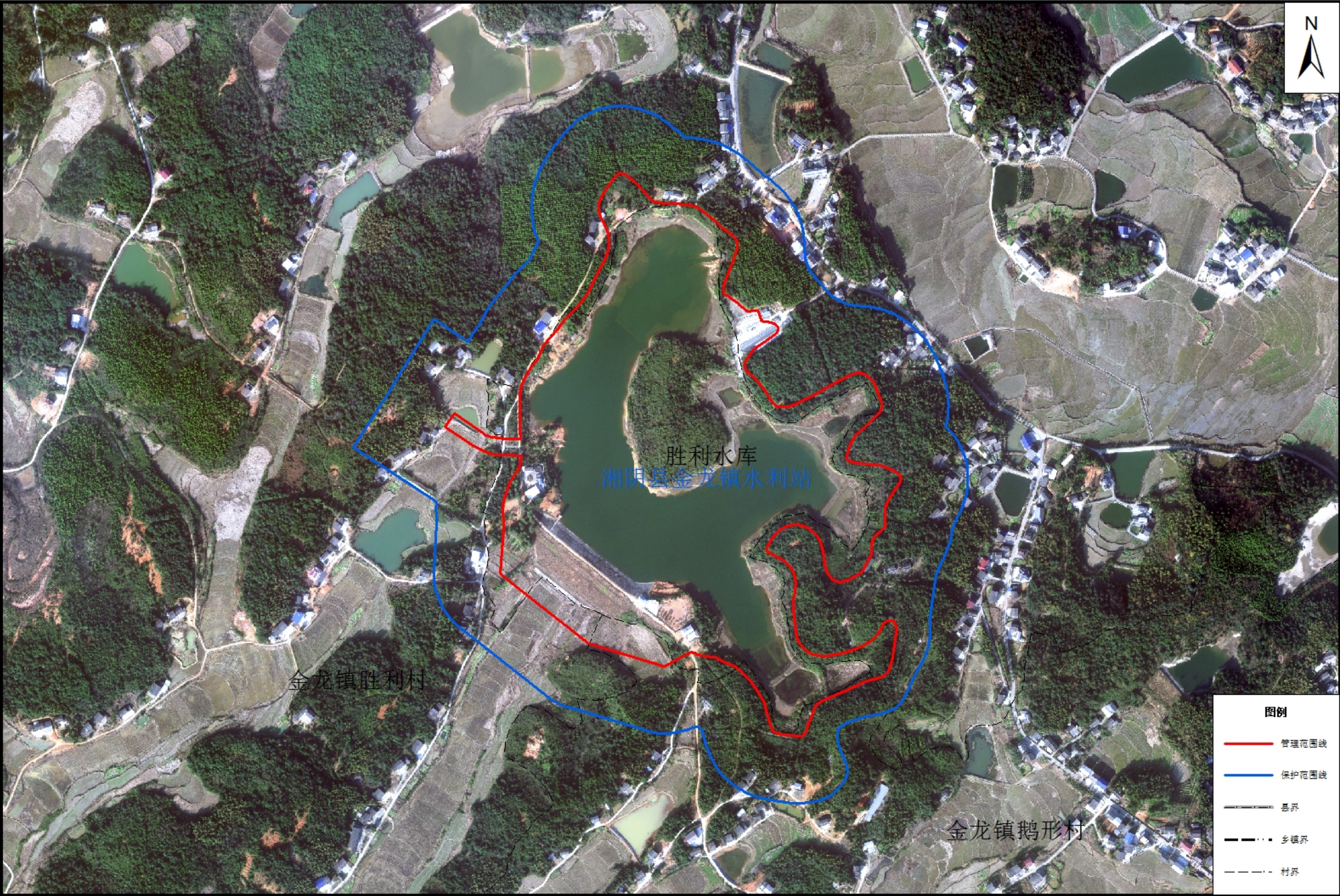
胜利水库管理与保护范围划界成果示意图
