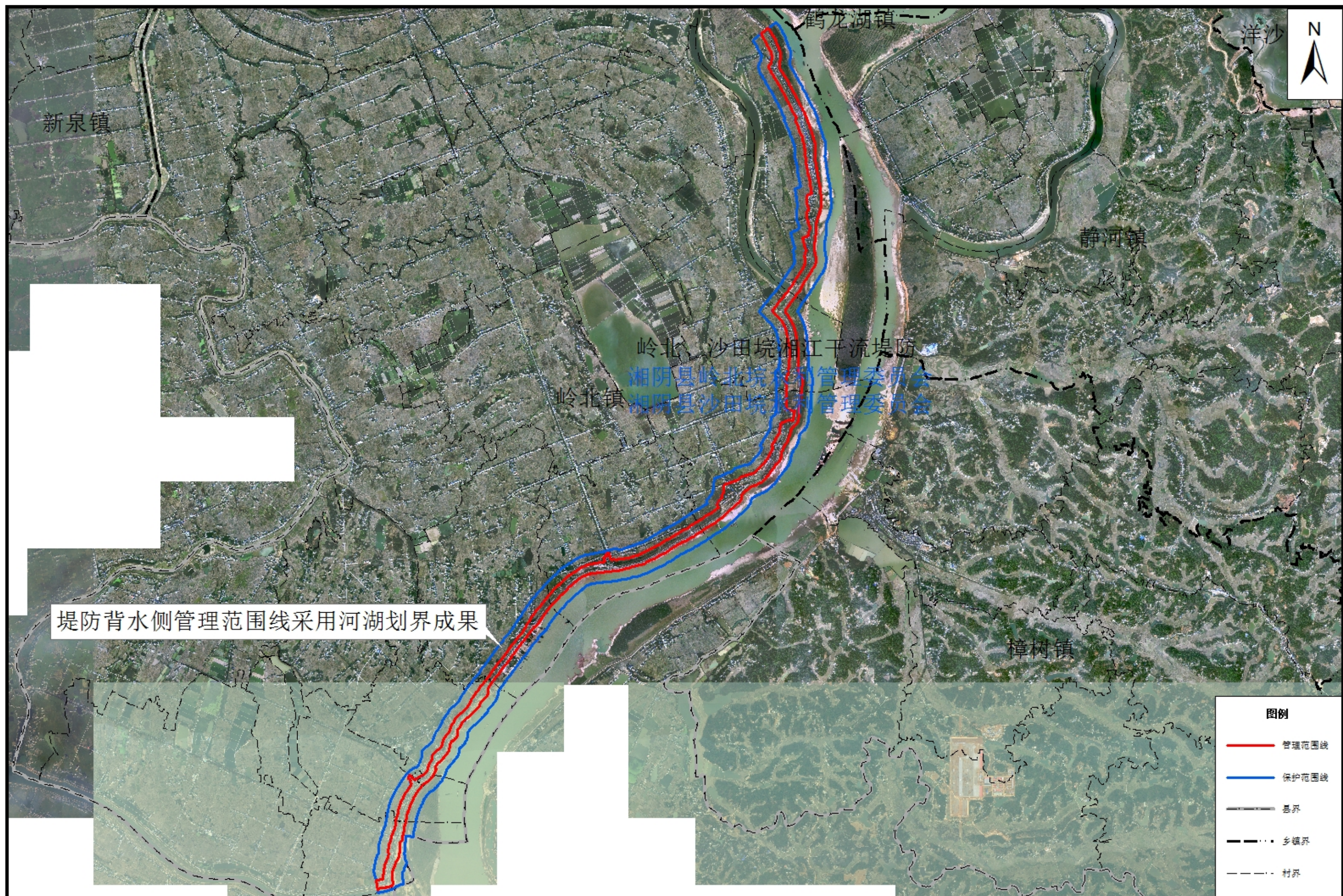
岭北、沙田垸湘江干流堤防管理与保护范围划界成果示意图
