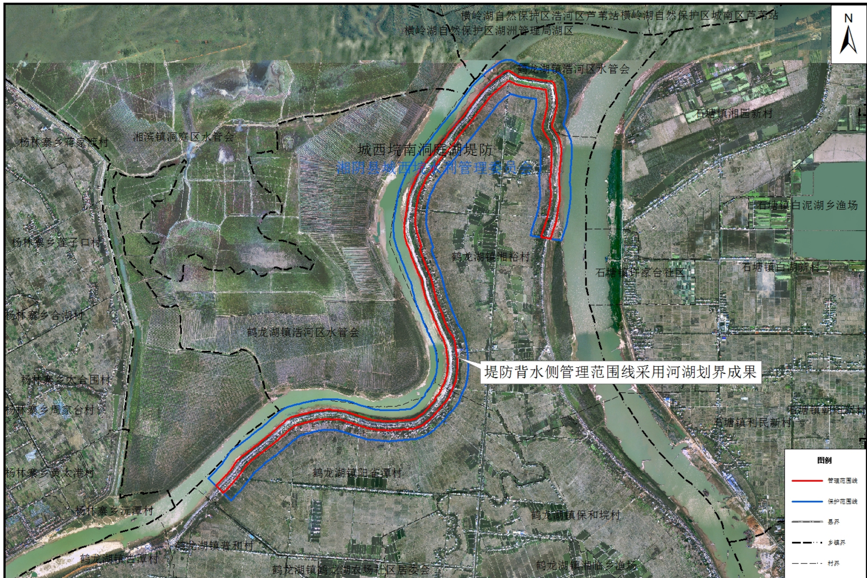
城西垸南洞庭湖堤防管理与保护范围划界成果示意图
