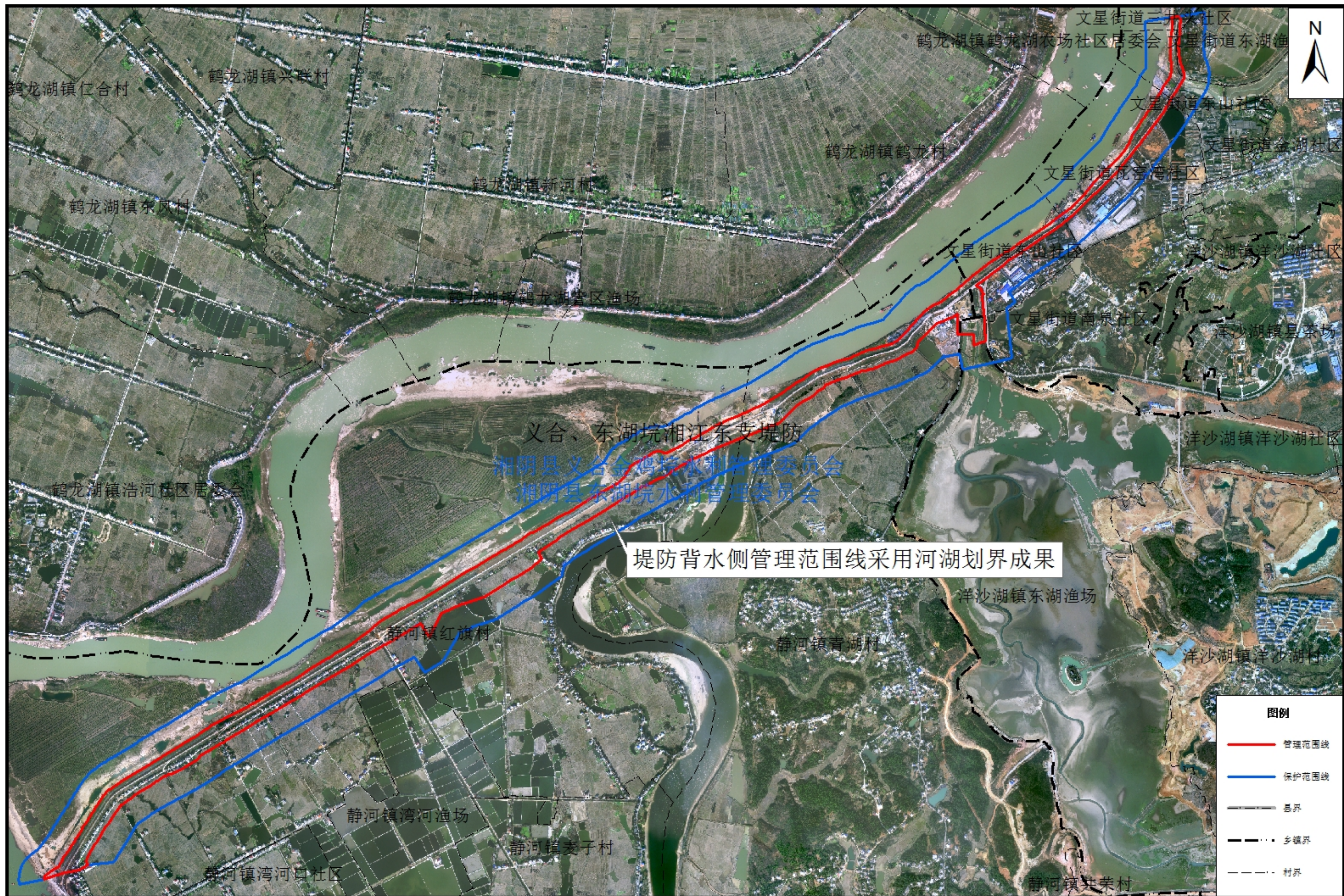
义合、东湖垸湘江东支堤防管理与保护范围划界成果示意图
