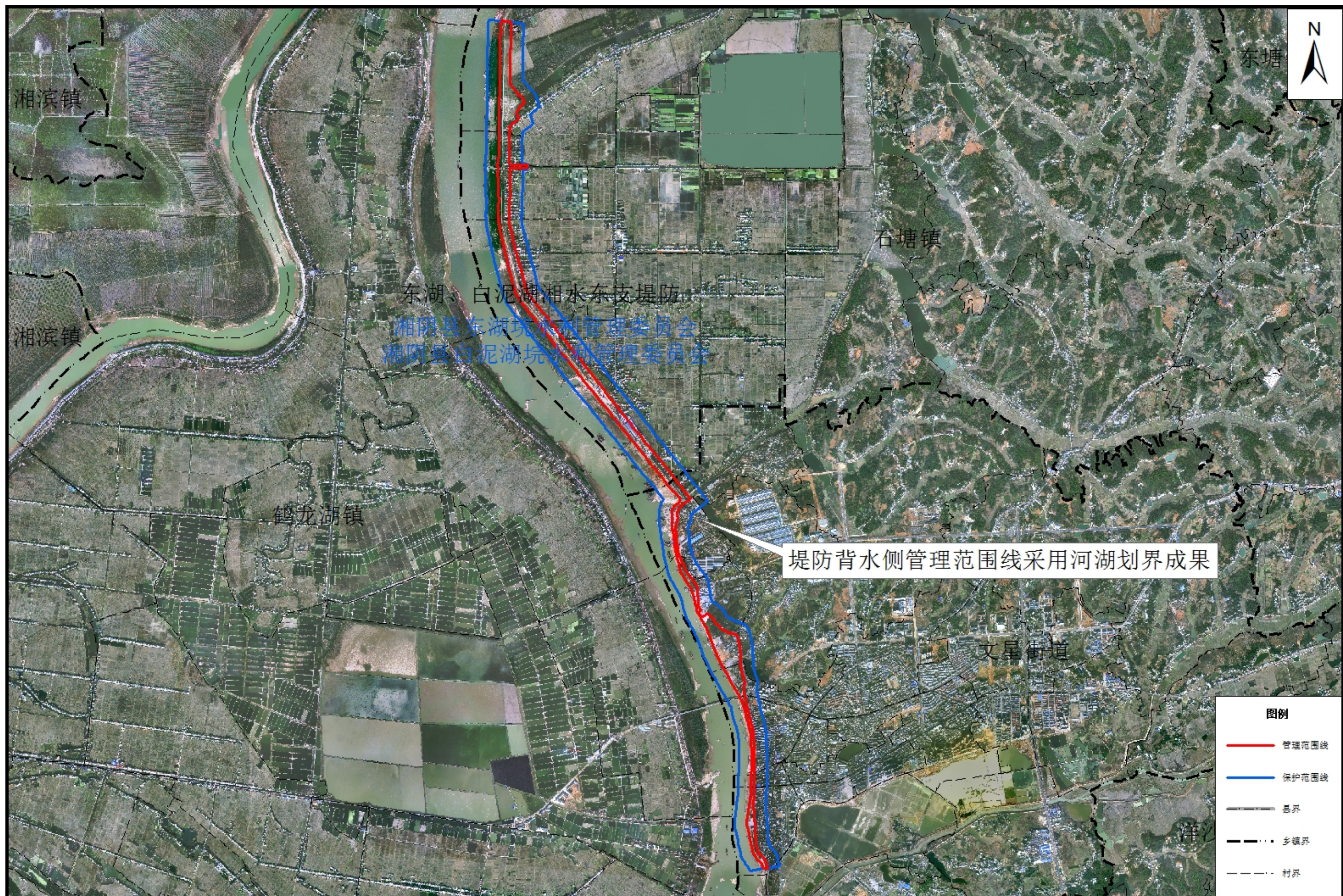
东湖、白泥湖湘水东支堤防管理与保护范围划界成果示意图
