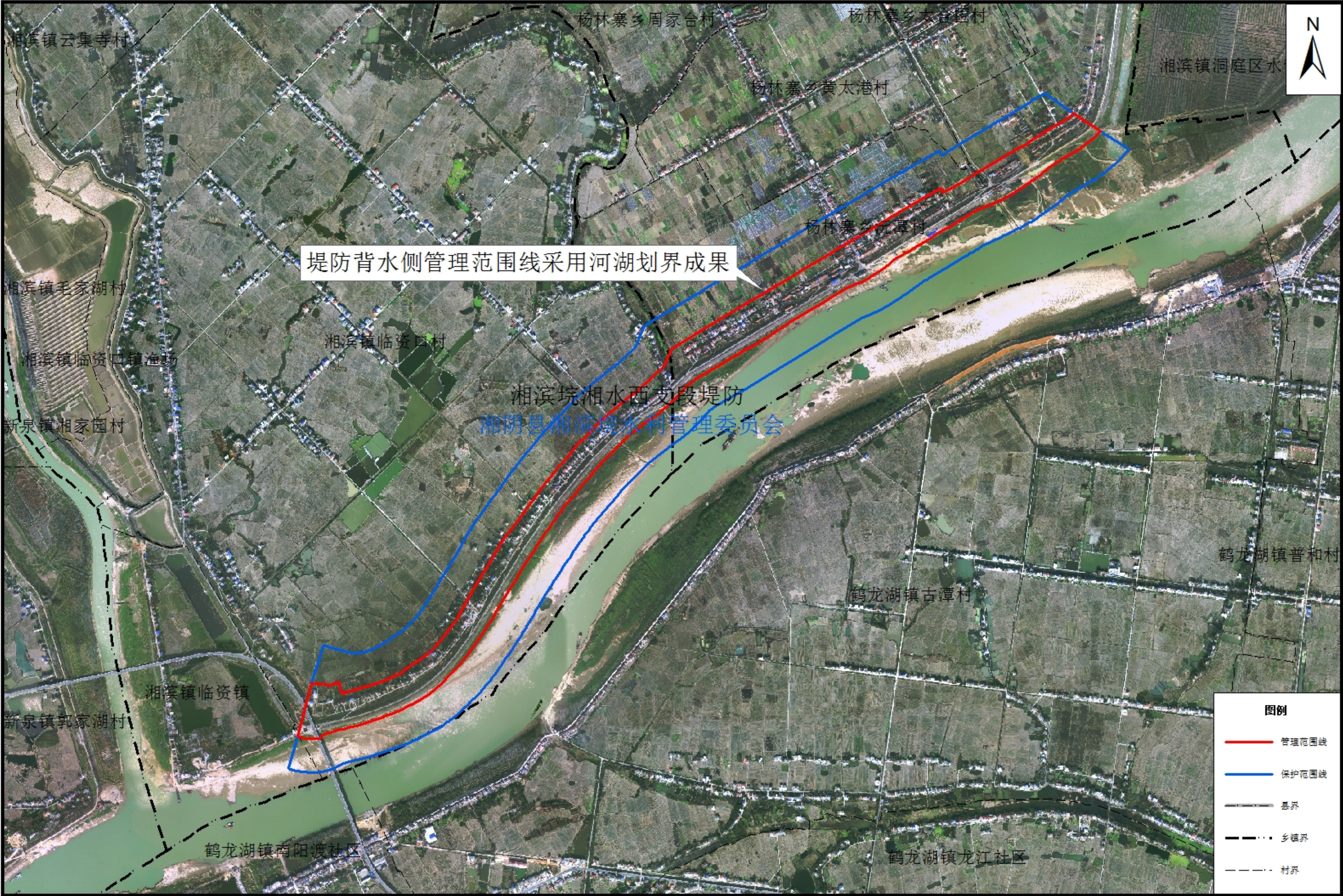
湘滨垸湘水西支段堤防管理与保护范围划界成果示意图
