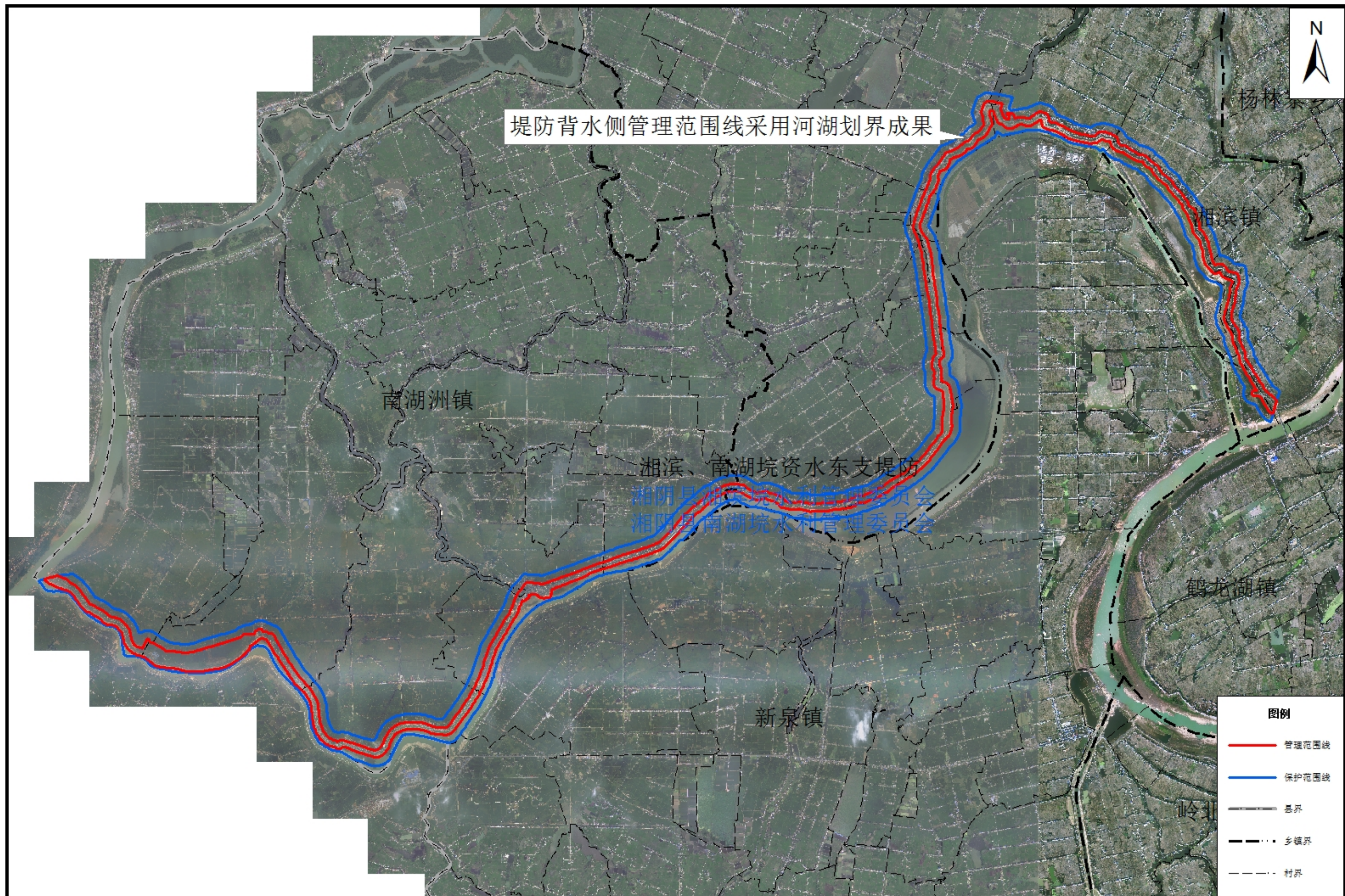
湘滨、南湖垸资水东支堤防管理与保护范围划界成果示意图
