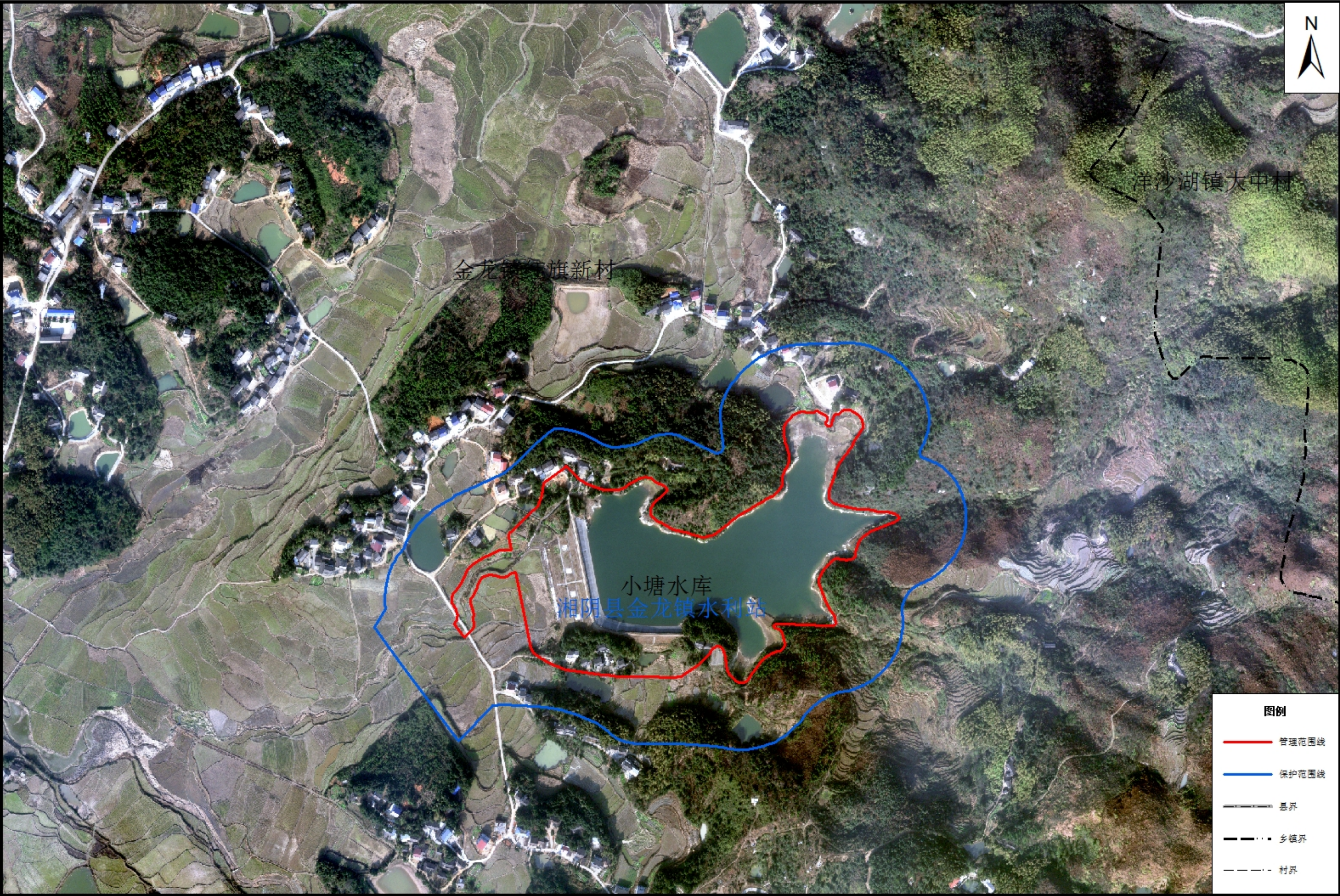
小塘水库管理与保护范围划界成果示意图
