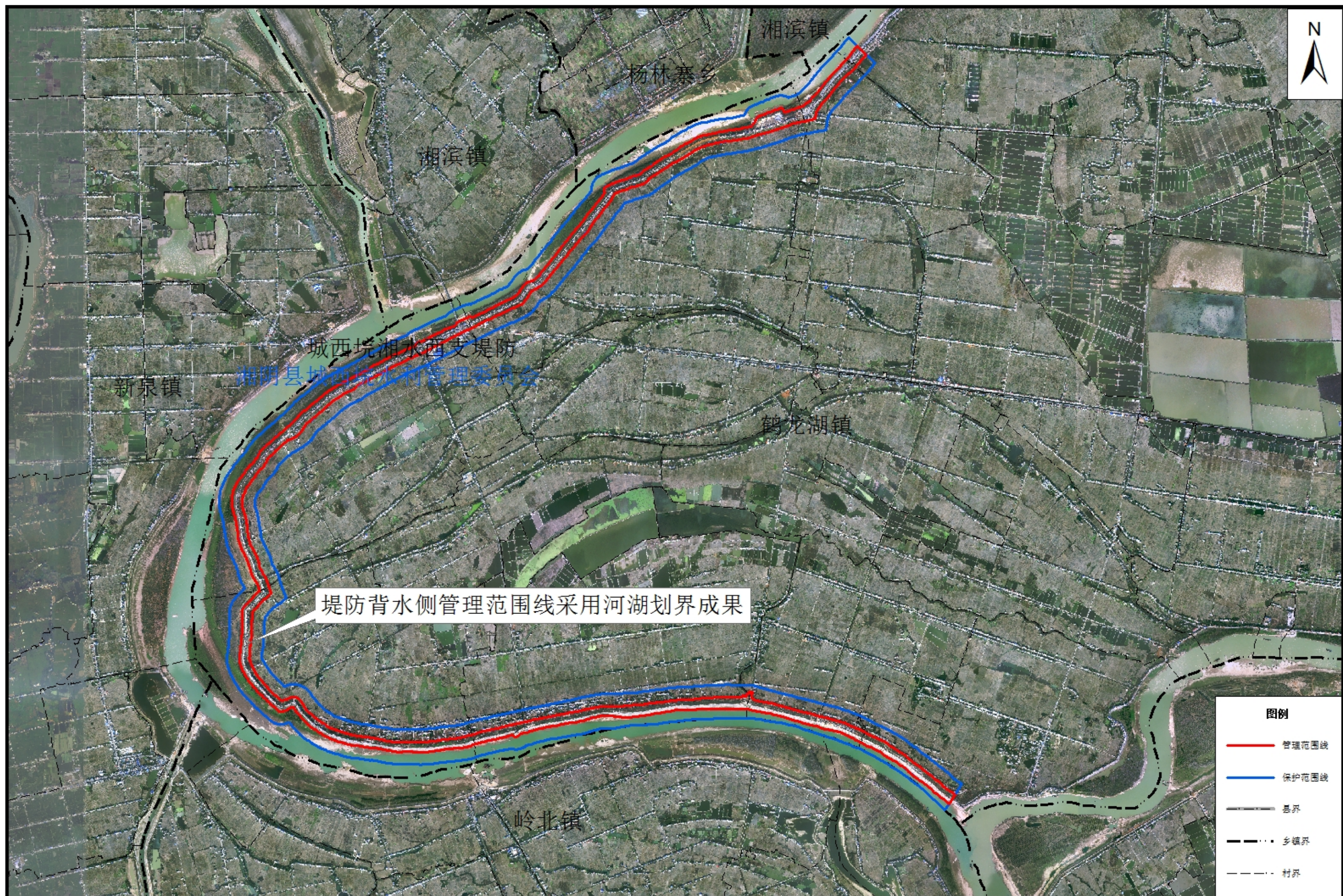
城西垸湘水西支堤防管理与保护范围划界成果示意图
