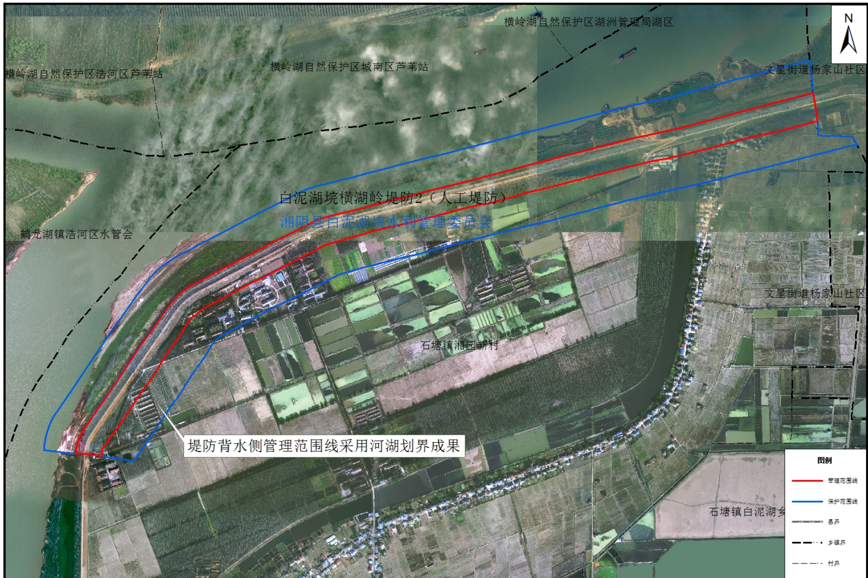
白泥湖垸横湖岭堤防2（人工堤防）管理与保护范围划界成果示意图
