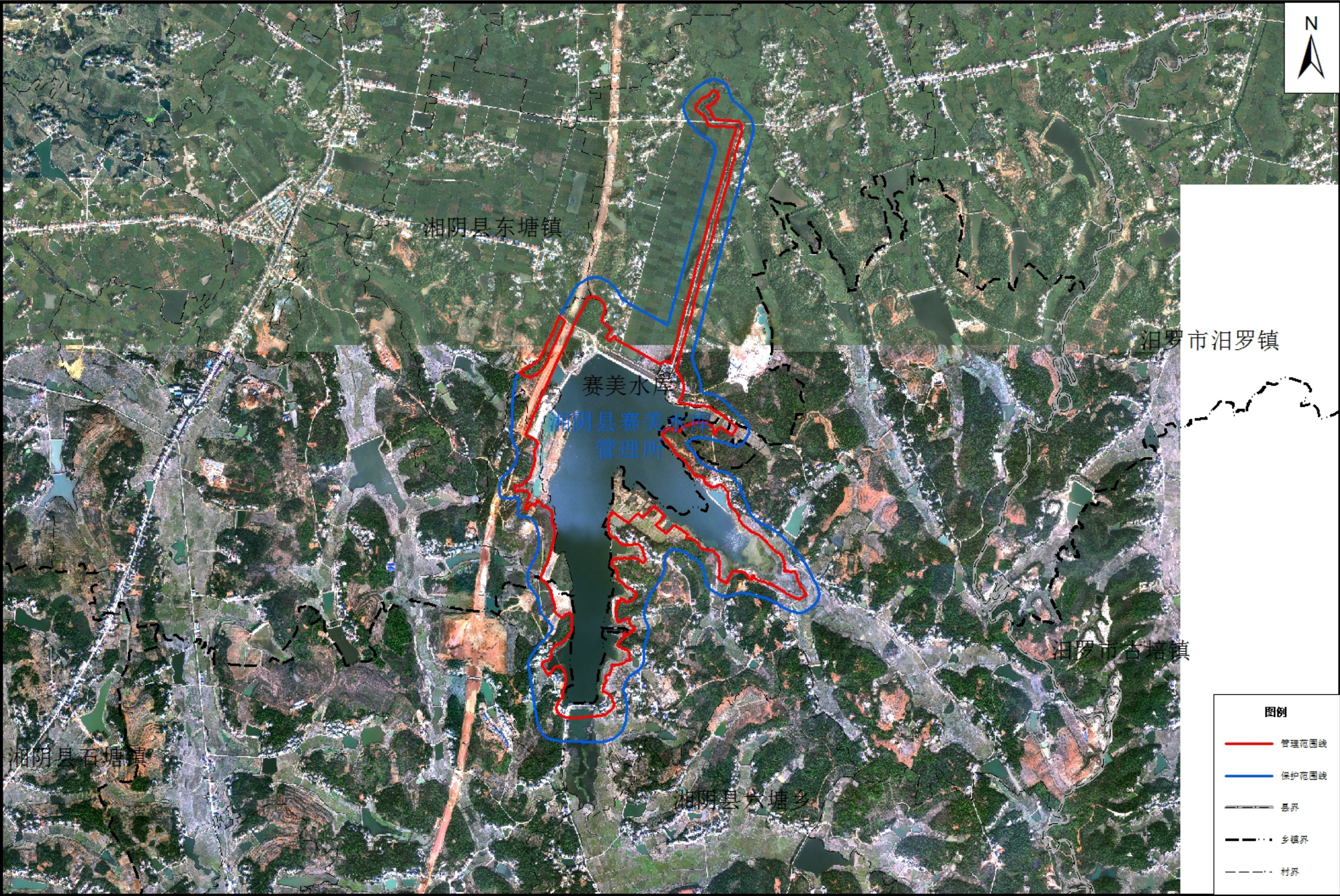
赛美水库管理与保护范围划界成果示意图
