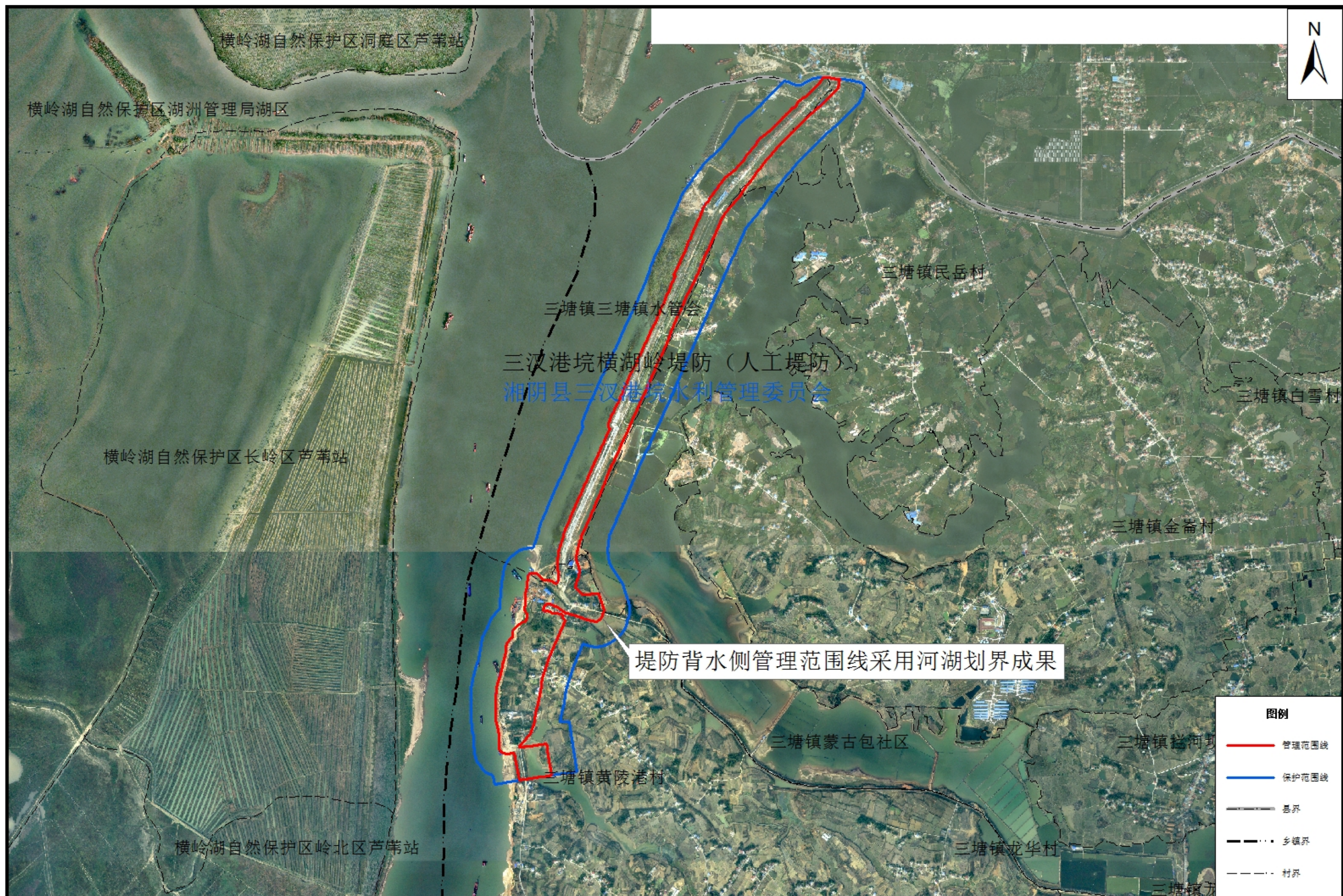
三汊港垸横湖岭堤防（人工堤防）管理与保护范围划界成果示意图
