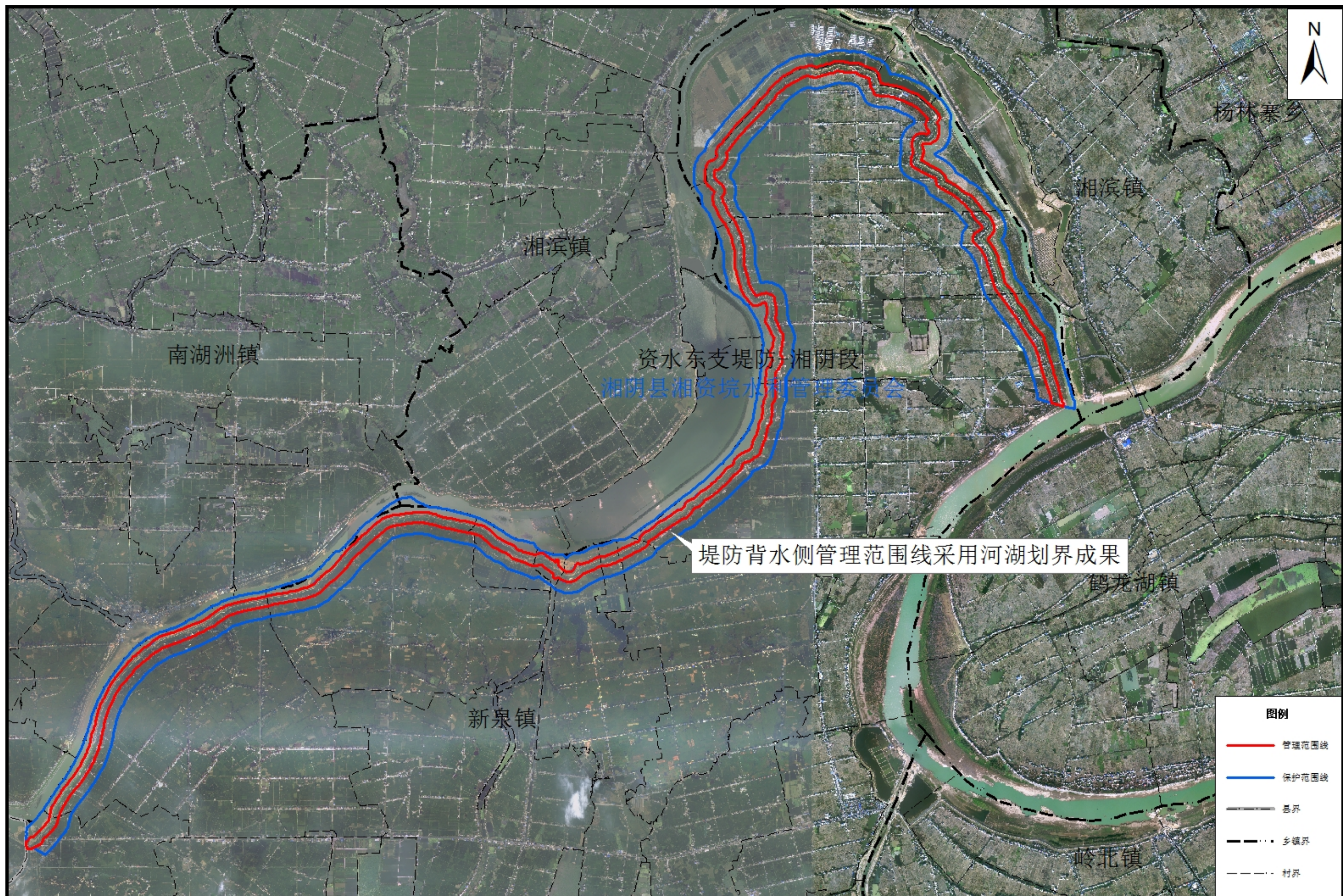
资水东支堤防-湘阴段管理与保护范围划界成果示意图
