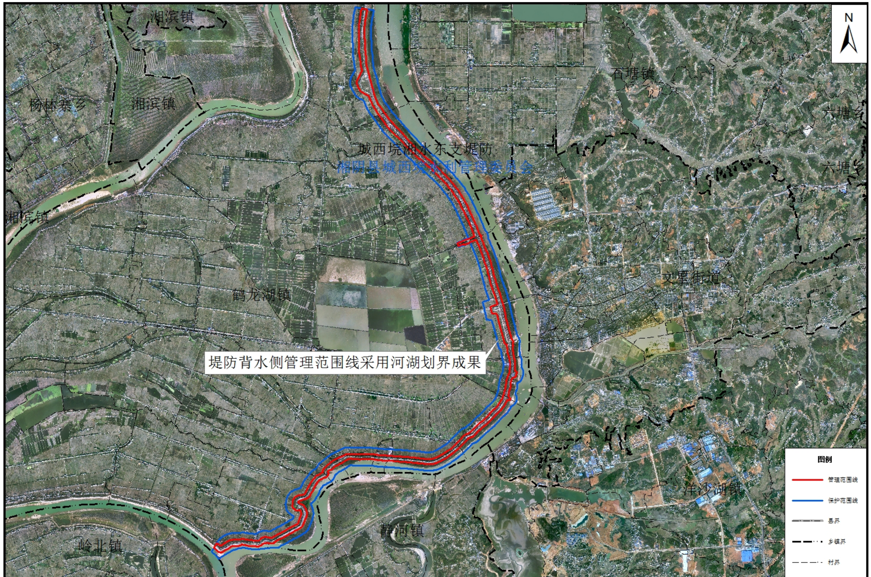
城西坑湘水东支堤防管理与保护范围划界成果示意图
