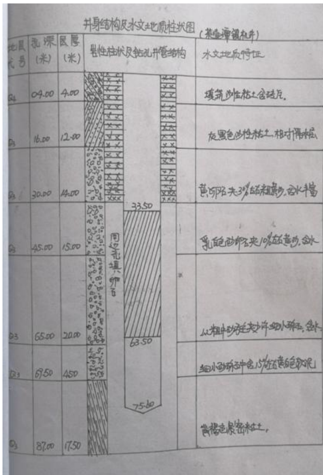
图 2-5 钻孔柱状图和成井工艺图
