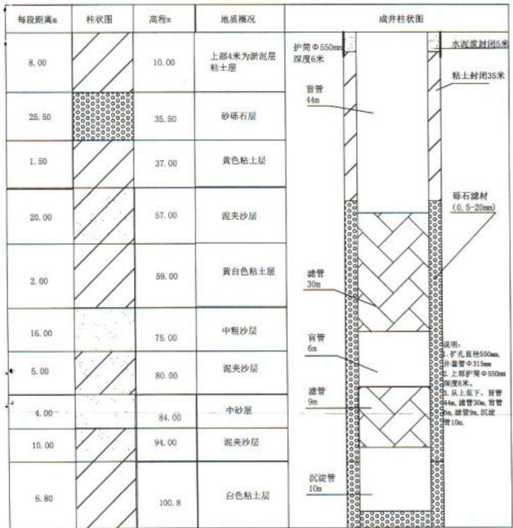
图 2-5 水井钻孔柱状图和成井工艺图
