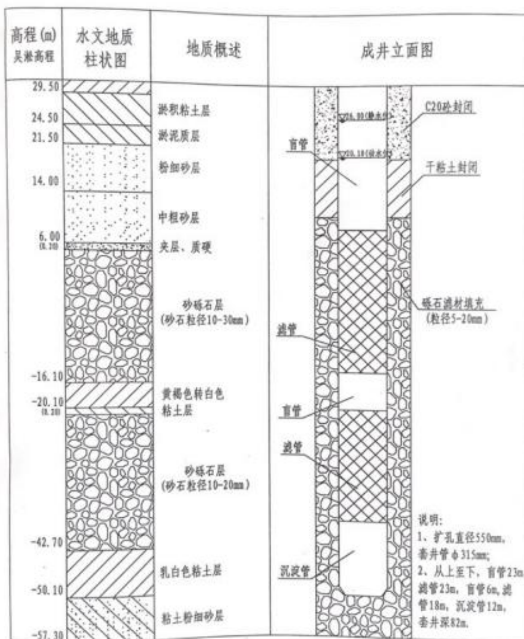
图 2-5 钻孔柱状图和成井工艺图
