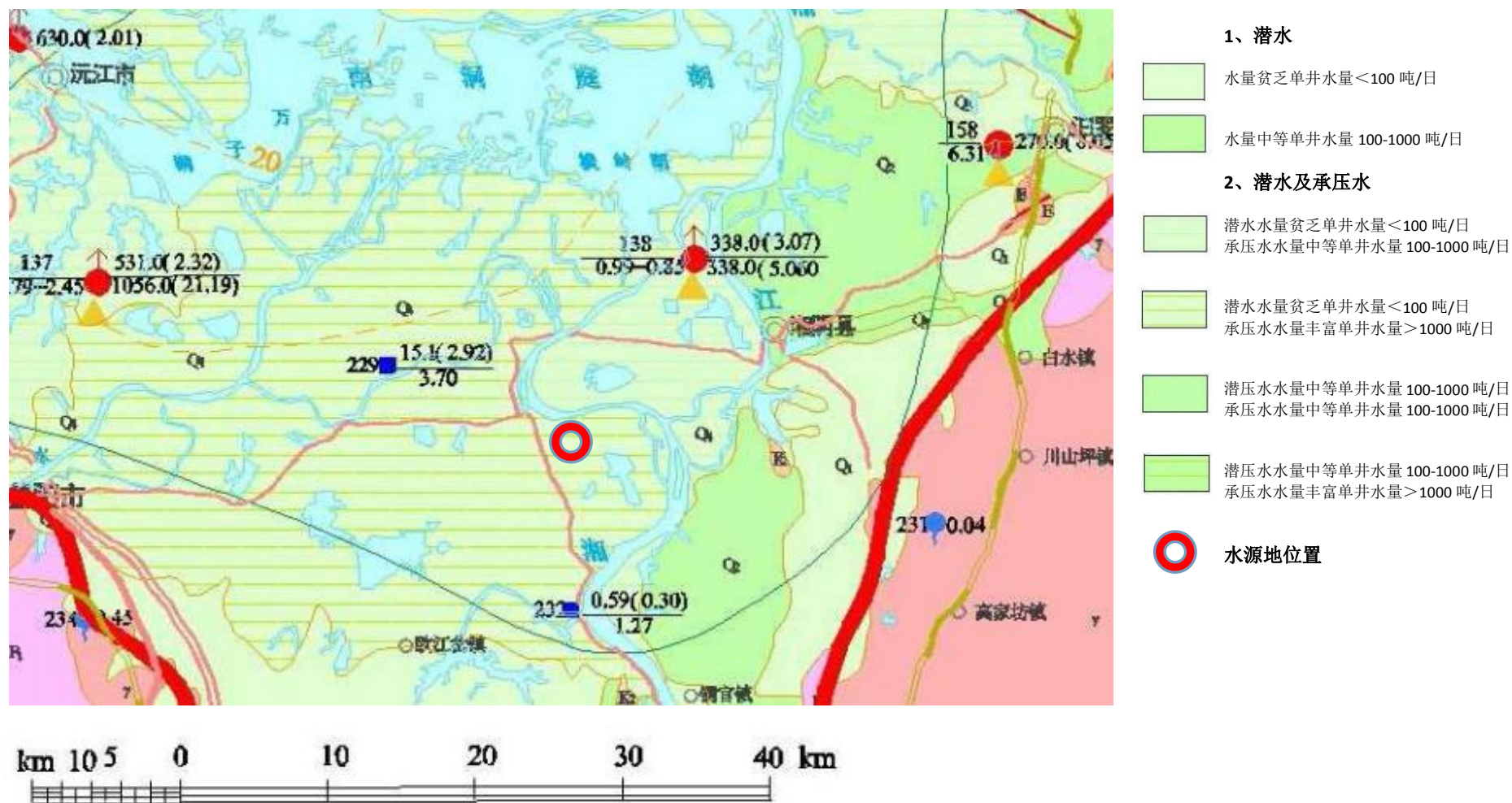
图 2-4 洞庭湖区水文地质图
