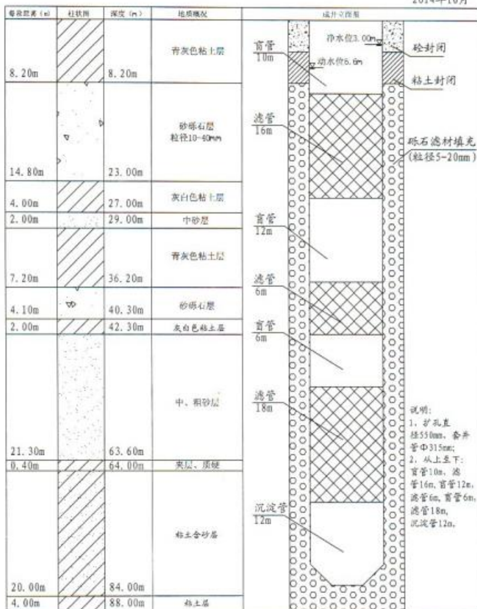
图 2-5-2 2#钻孔柱状图和成井工艺图
