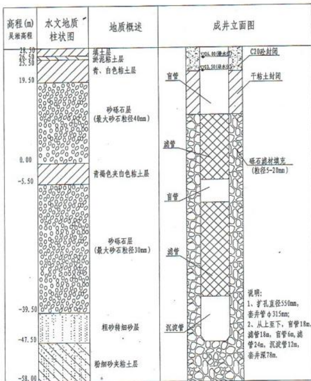
图 2-5-1 1#钻孔柱状图和成井工艺图
