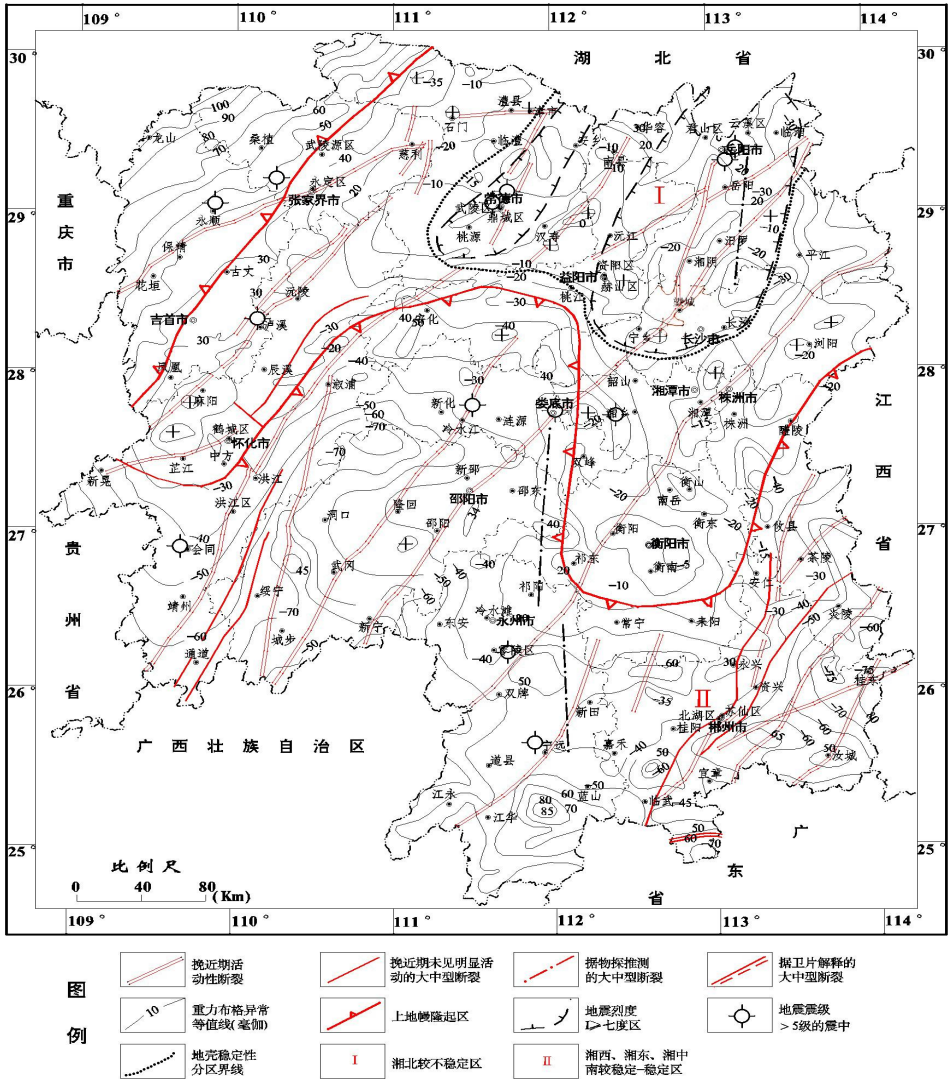
图 1 工作区中的地形地貌图及构造、地质控制条件
