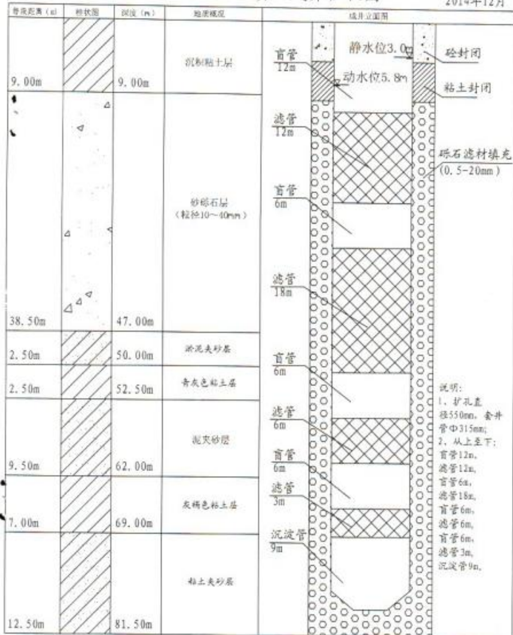
图 2-5-2 2 号井钻孔柱状图和成井工艺图 (b)
