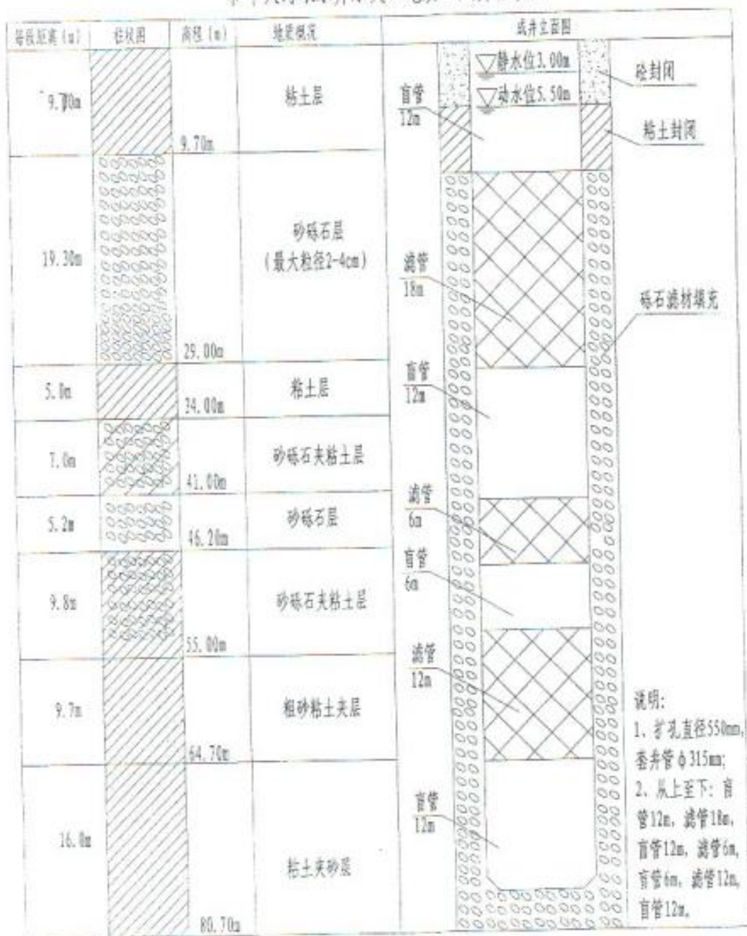
和平大湾取水井水文、地质、成井柱状图
