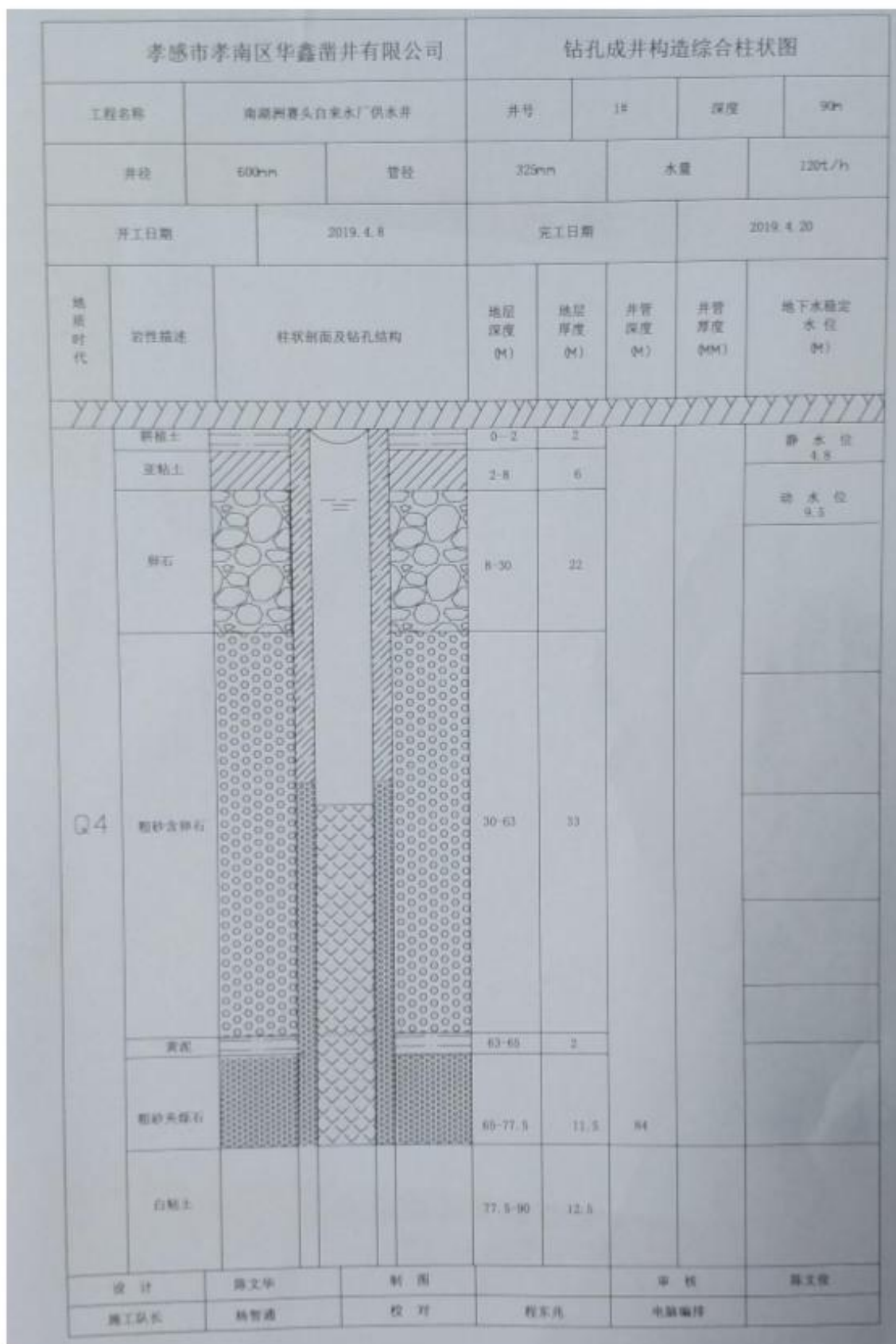
图 2-5 钻孔柱状图和成井工艺图
