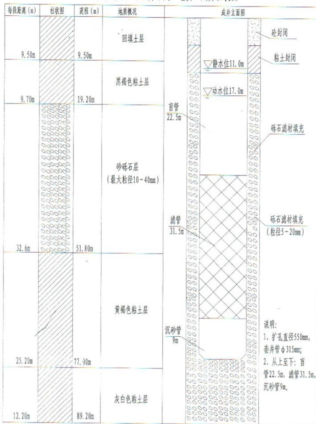
和平闸水厂取水井水文、地质、成井柱状图
