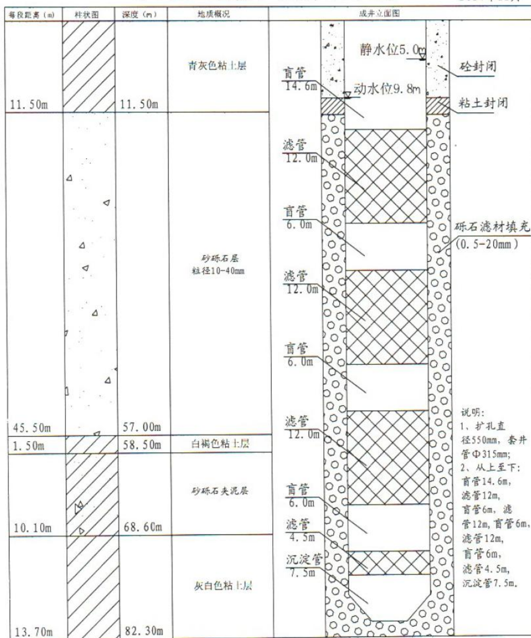
图 2-5-2 2#井钻孔柱状图和成井工艺图
