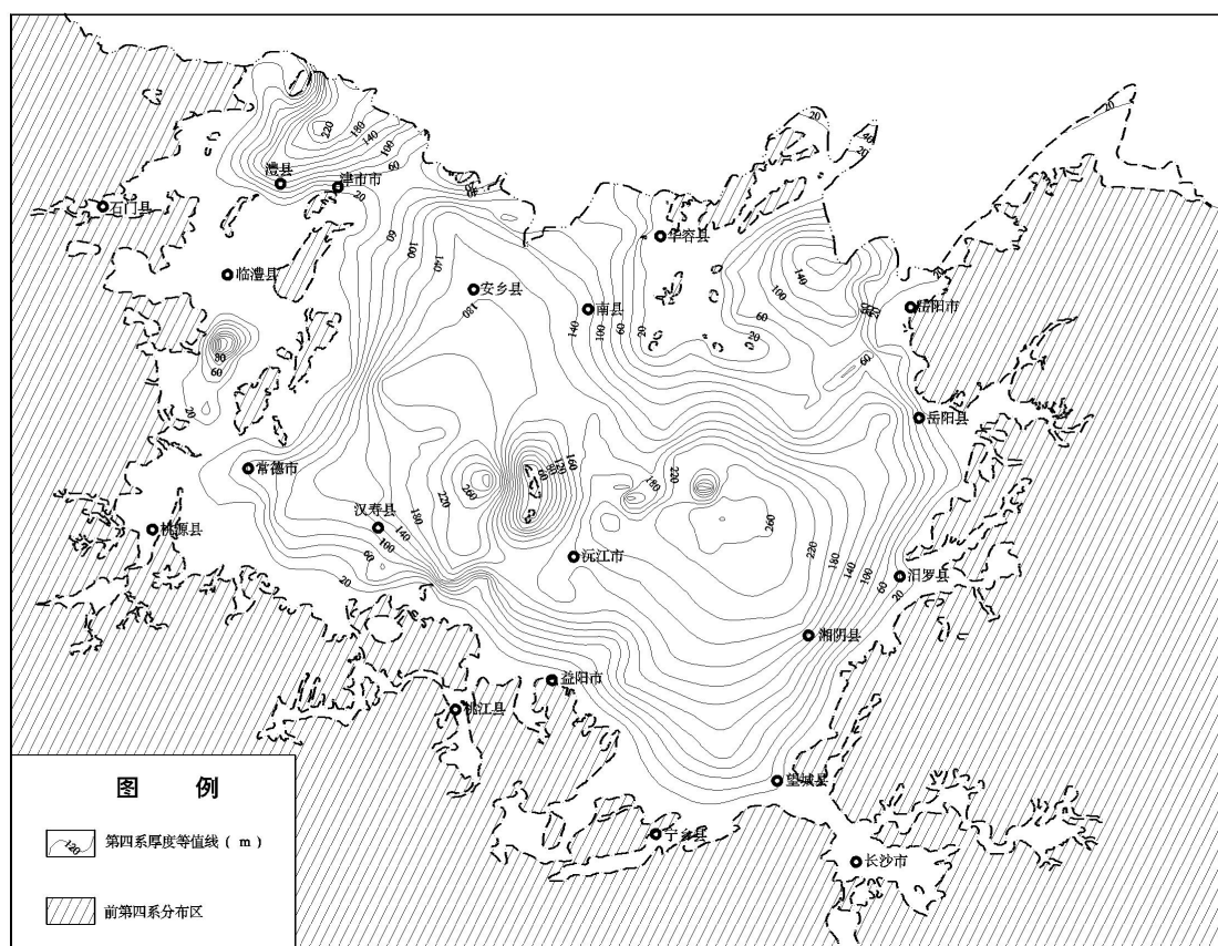
图 2-2 洞庭湖区第四系沉积厚度等值线图
