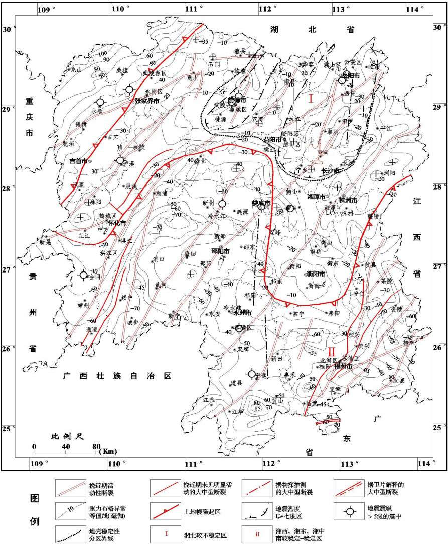
图 2-3 湖南省构造及地壳稳定性图
