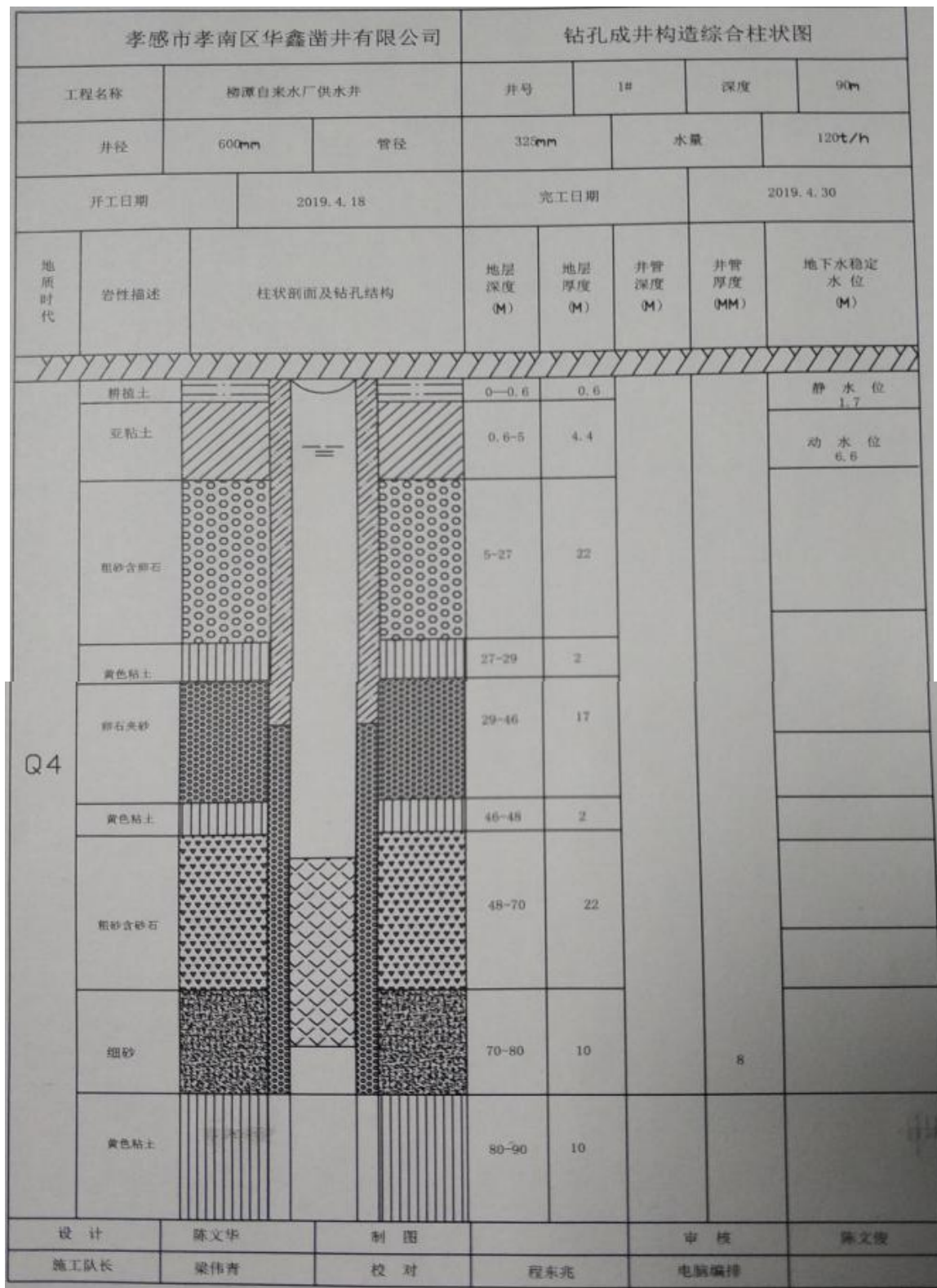
图 2-5 钻孔柱状图和成井工艺图
