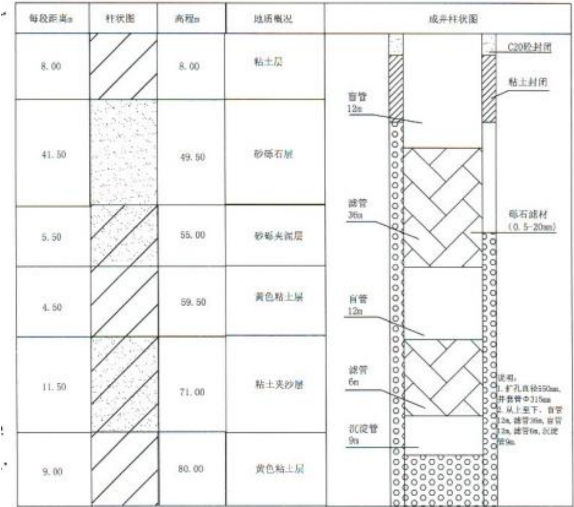
图 2-5 2#钻孔柱状图和成井工艺图
