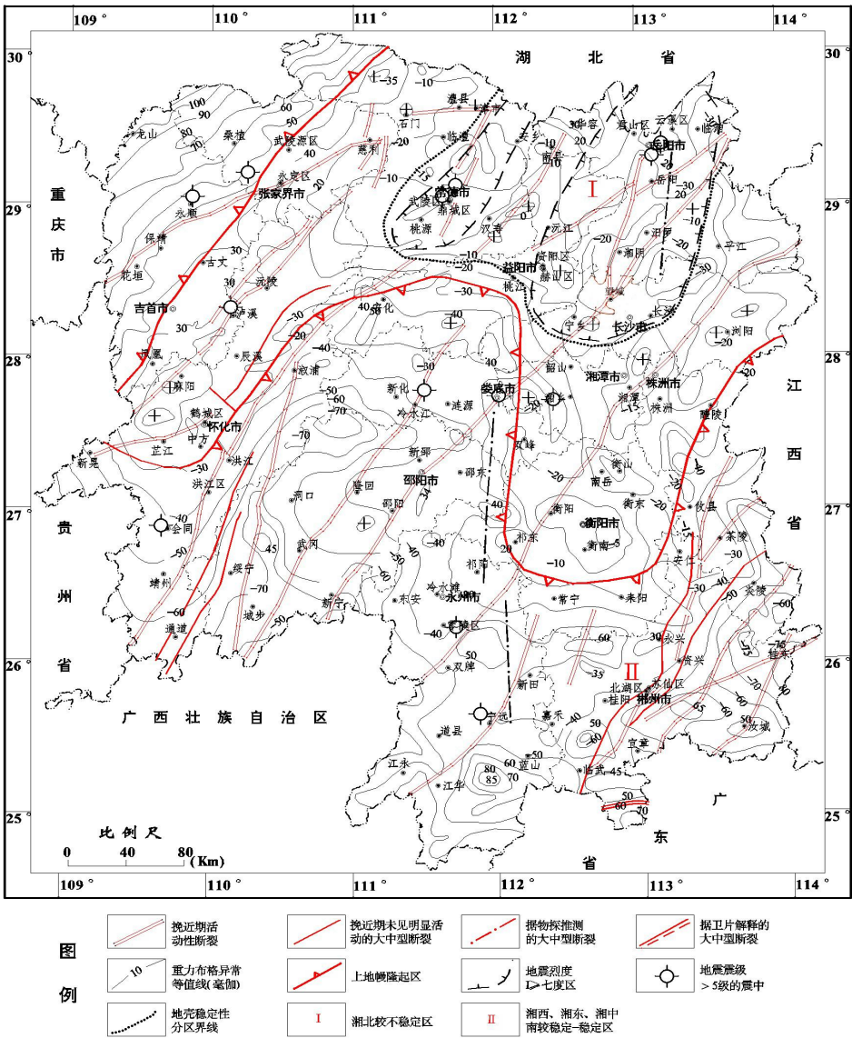
图 2-3 湖南省构造及地壳稳定性图
