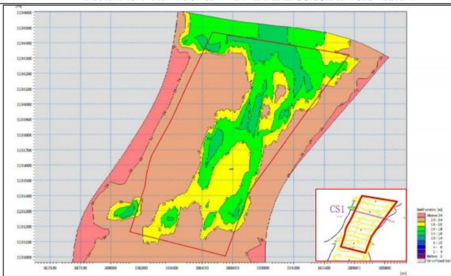
图2.1-5 项目区北段河床高程分布图
