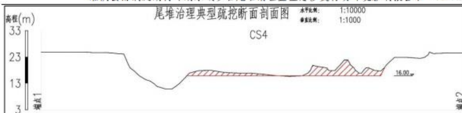
图2.1-7 项目区典型断面治理剖面示意图
