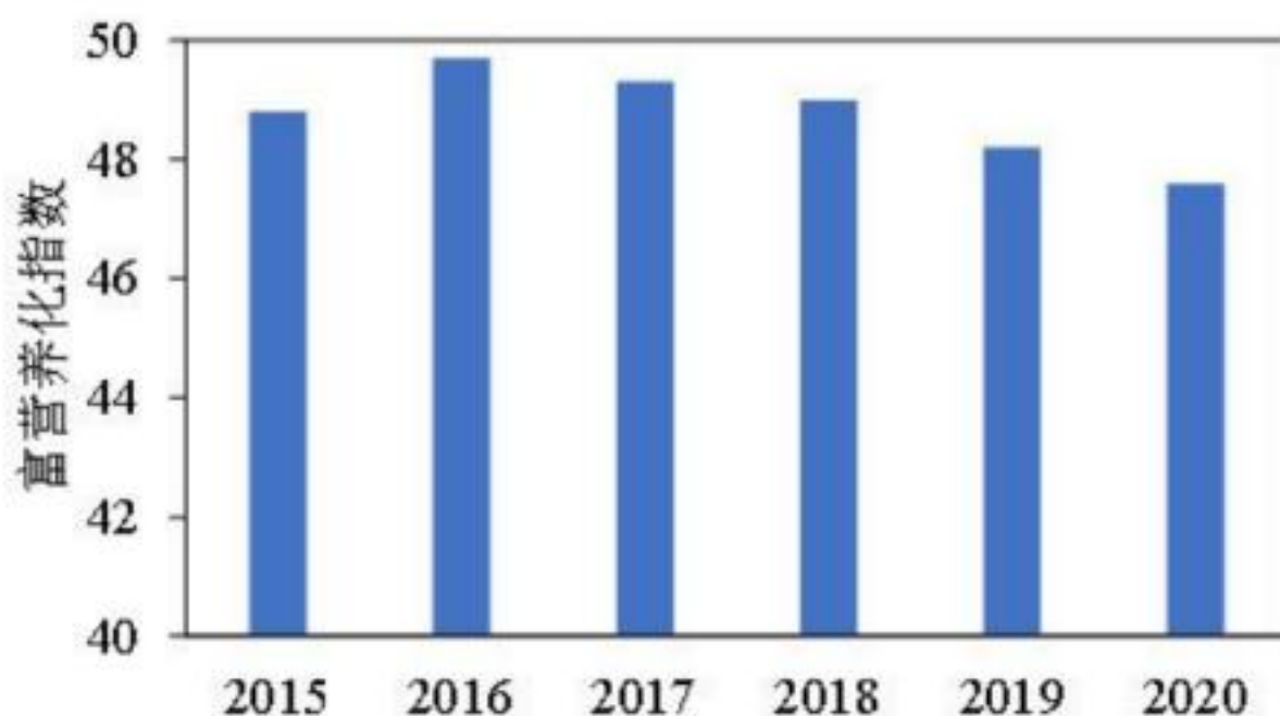
图3.4-2 洞庭湖水体富营养指数变化图
