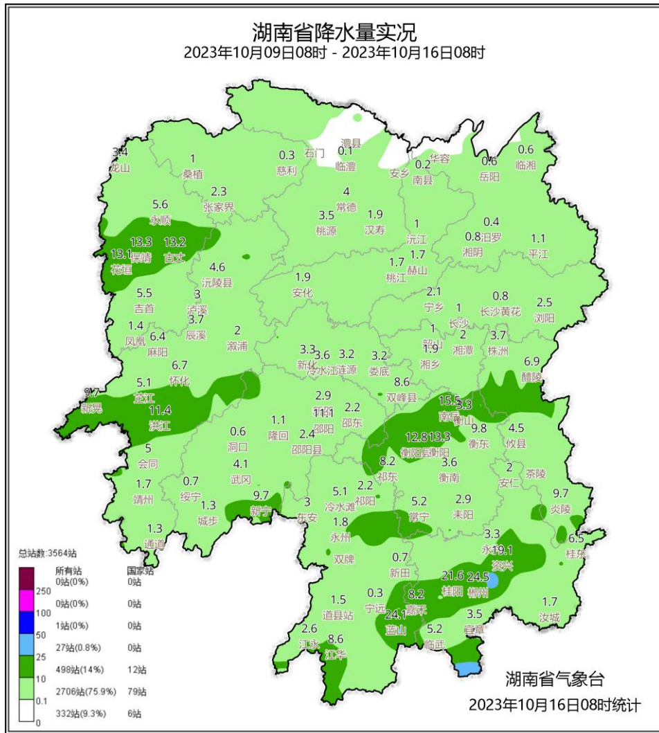
附图1 湖南降雨量实况(10月9日08时至16日08时)
