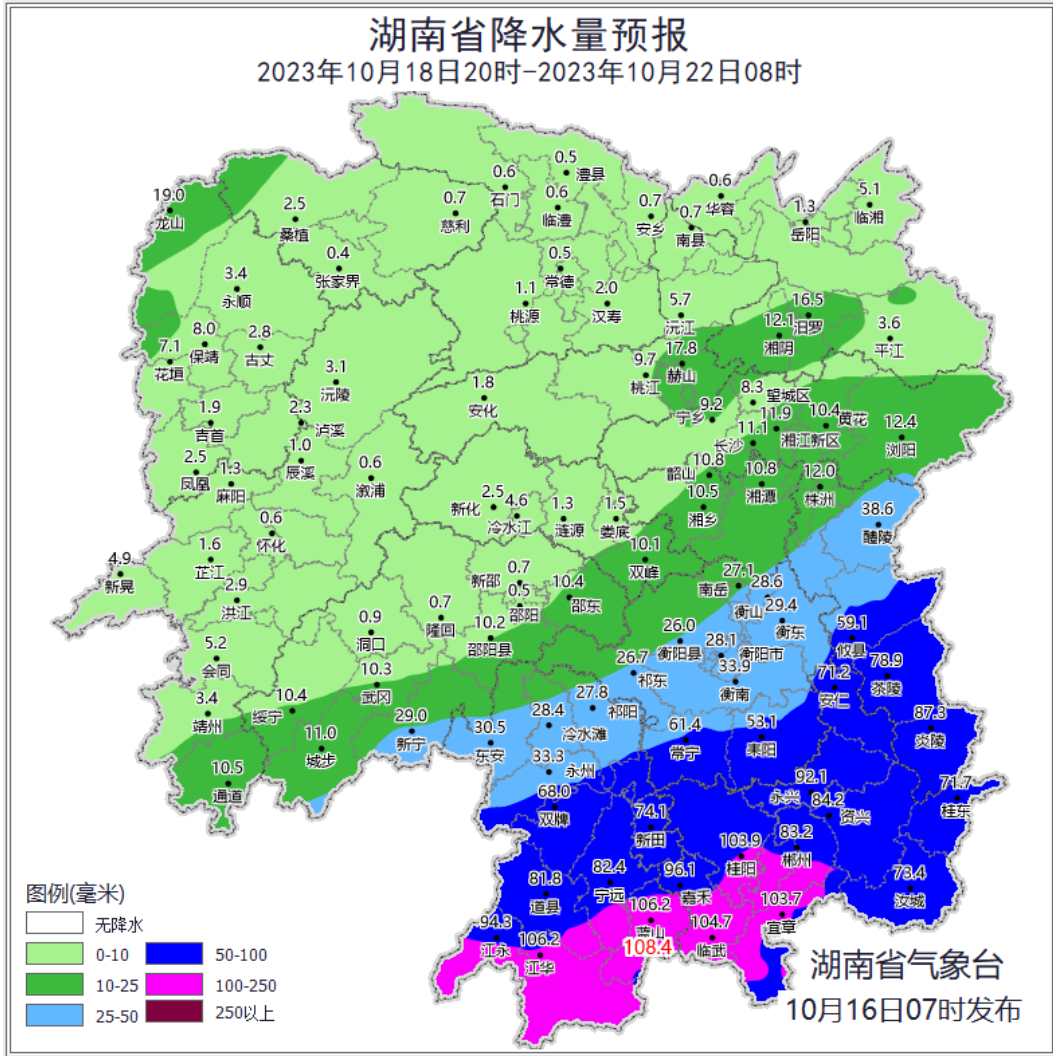
附图3 湖南累计降雨量预报(10月18日20时至22日08时)
