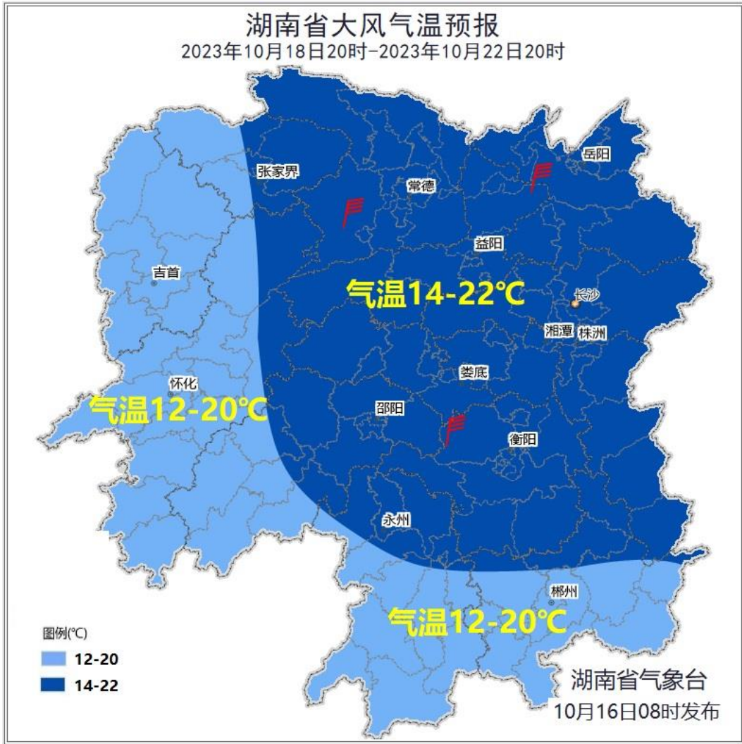
附图2 湖南省大风气温预报(10月18日20时至22日20时)
